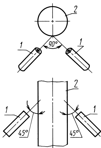
1 — горелка; 2 — образец
