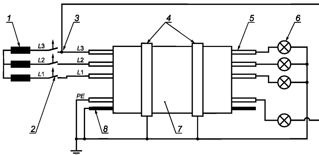
1 — трансформатор; 2 — плавкий предохранитель (2 А); 3 — подсоединение к линии L3 (или L1 , или L2 ); 4 — поддерживающие кольца; 5 — испытательная жила или группа жил; 6 — нагрузочный индикаторный прибор (например, лампа); 7 — образец; 8 — металлический экран (если имеется); L1 , L2 , L3 — линии испытываемых жил или групп жил ( L2 , L3 , если имеются); PE — жила заземления (если имеется)
