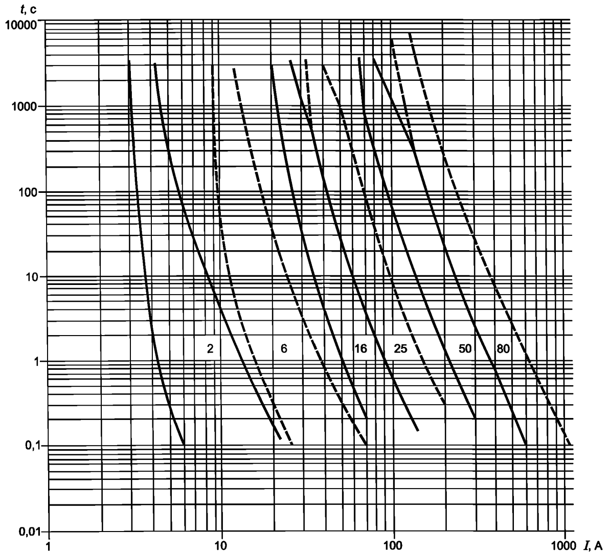
Рисунок А.1 — Время-токовые зоны для плавкого предохранителя
