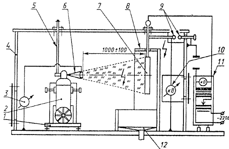
Рисунок 1 – Принципиальная схема испытательного стенда определения тока утечки по струе заряда огнетушителя.
